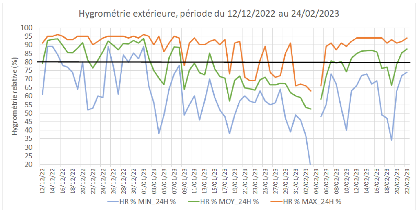
Figure 2 : Humidité relative extérieure
